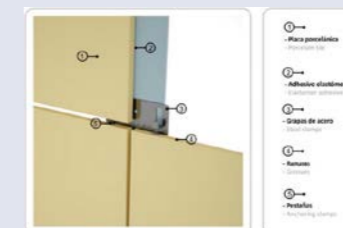
GRAPA OCULTA HIDDEN CLIPS
